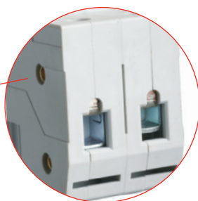
高接线端子能力 25mm 2 or 2 × 10mm 2 for MCB's 可连接叉型汇流排
